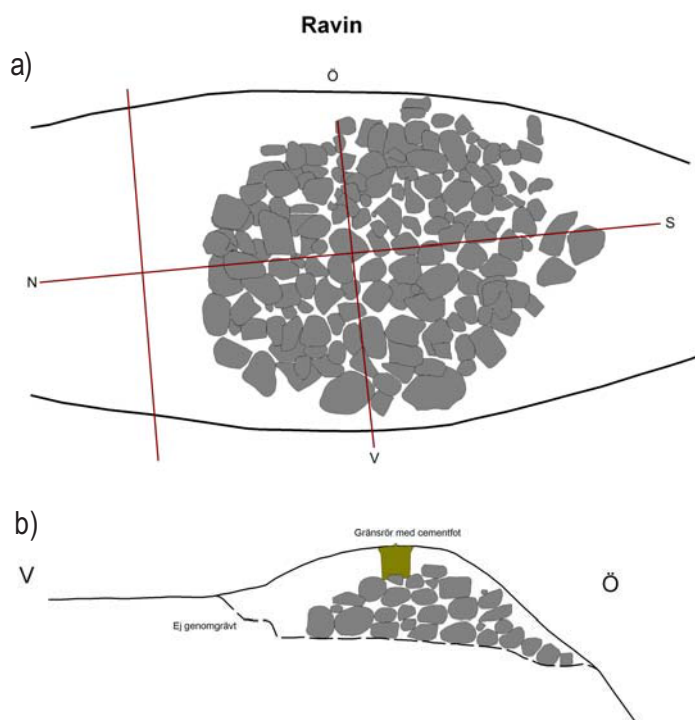
Fig. 13a-b. Plan (a) och profil (b) av grav XIII i Skyttberg. Digitaliserat från Cajmats ritning av författaren.
